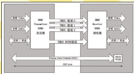
● HDMI 接口工作原理
