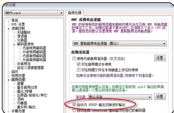
●图 5 启用 SPDIF 功能
