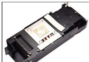
● 加强设计的散热系统
