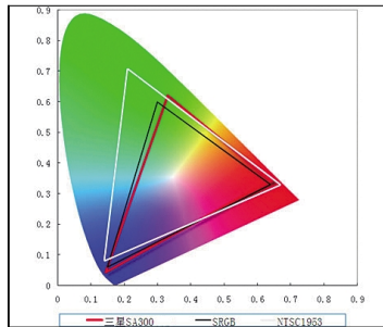
● SA300 的色域涵盖了 sRGB 的 74.3%,是同档次中相当出色的一款产品
