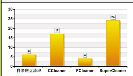
扫描垃圾文件耗时对比 (单位:秒,数值越小越好)
