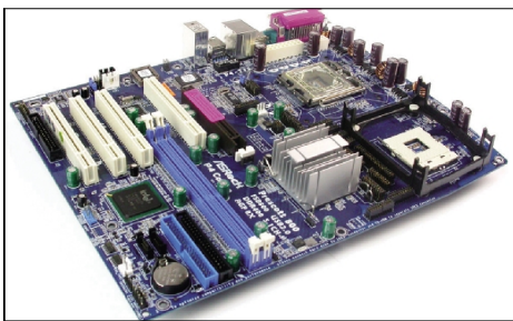
● 华擎 P4 COMBO 提供了两个不同的处理器接口
