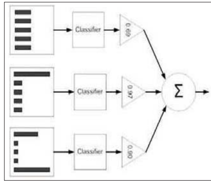
基于Boost原理的混合分类算法模型原理
