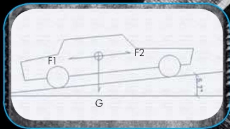
图3-2 坡道定点停车和起步模型图
