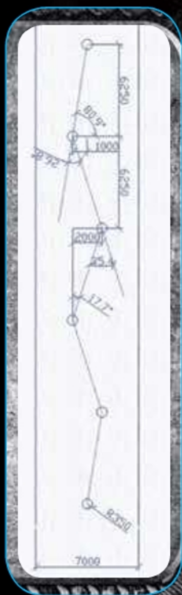
图8-2 穿桩考试模型图
