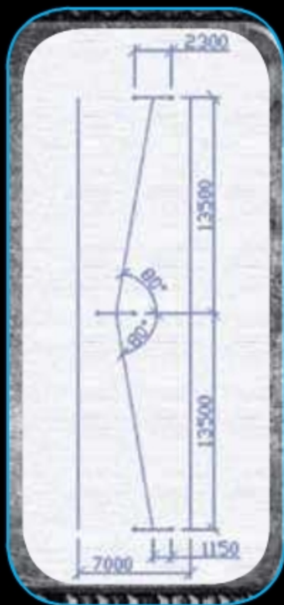
图5-3 限速通过限宽门模型图
