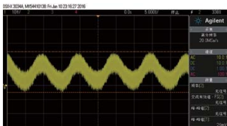
Tt SMART DPS G 12V/40A工频纹波
