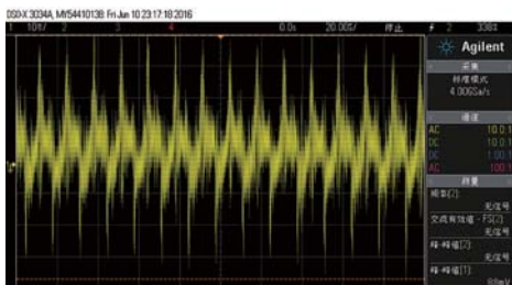
Tt SMART DPS G 12V/40A开关纹波
