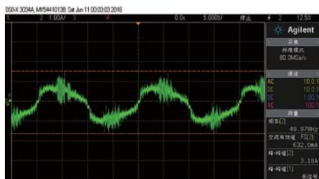
■ 银欣SST-ST75F-PT 12V/10A输入电流波形
