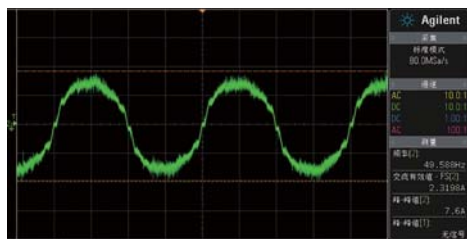
■ 银欣SST-ST75F-PT 12V/40A输入电流波形
