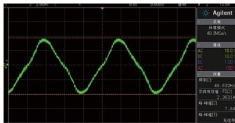
■ Tt SMART DPS G 12V/40A输入电流波形
