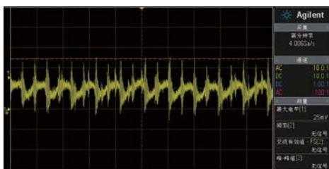
银欣SST-ST75F-PT 12V/40A开关纹波
