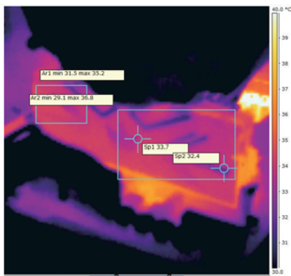
■ 影驰名人堂DDR4 4000的内存散热片性能表现优异, 在DDR4 4000四个小时的烤机测试中, 其散热片表面平均温度不到40°C。
