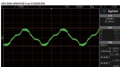
■ 游戏悍将魔尊GP700M特效版12V/10A输入电流波形
