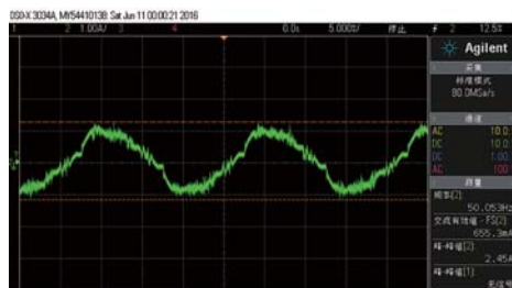
■ 海盗船RM750x 12V/10A电流输入波形
