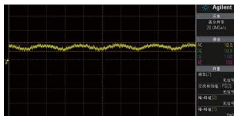
海盗船RM750x 12V/40A工频纹波
