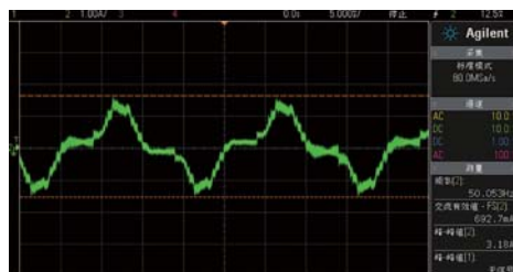
■ 安耐美赤焰金魔12V/10A输入电流波形
