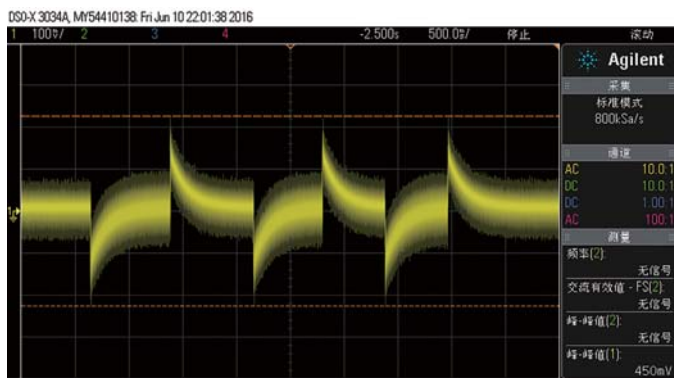
■大水牛金牛800负载跳变
