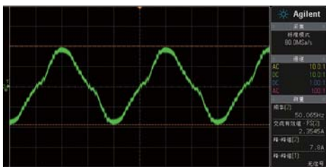
■ 游戏悍将魔尊GP700M特效版12V/40A输入电流波形
