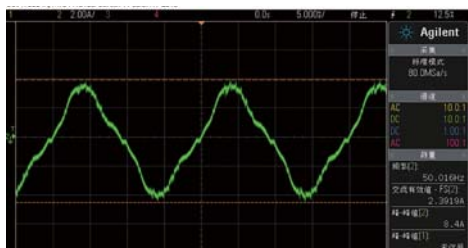
■ 大水牛金牛800 12V/40A输入电流波形
