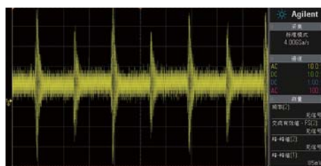
海盗船RM750x 12V/40A开关纹波
