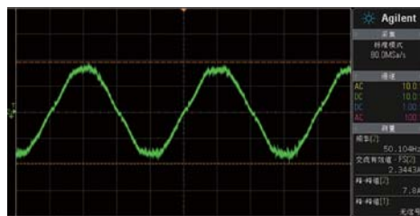
■ 海盗船RM750x 12V/40A电流输入波形
