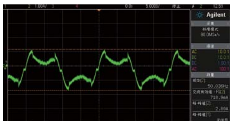
■ 大水牛金牛800 12V/10A输入电流波形
