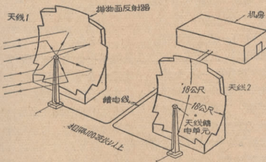
图3 天线的布置
