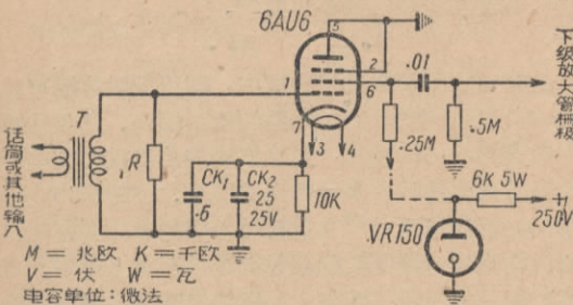
图1 低杂音输入放大器（增益约20）。R数值视变压器T比数及输入电路阻抗而定，约50—250千欧，不用输入变压器时，最高可至5兆欧。
