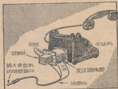
图5 自制电话检听器使用时情形
