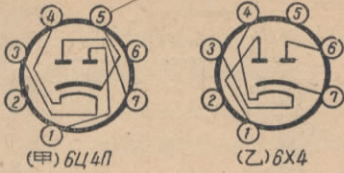
圖 2 6U4N 与 6X4 的管内电极接法
