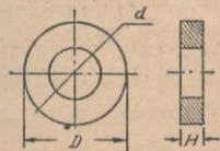
丙. 環形磁心 材料: 磁性瓷 1, 4, 5
