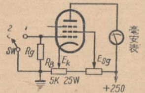
图2 测试电子管真空度优劣的简单线路。Rg的数值在测试功率管6V6、807、6L6等时约为0.5—1兆欧；测试一般电压放大管时约为1—5兆欧。
