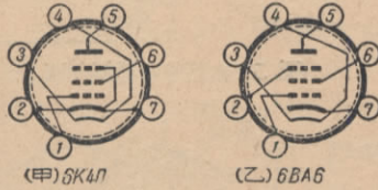
圖 3 6K4N 与 6BA6 的管内电极接法
