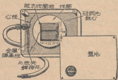
图3 电话检听器解剖图
