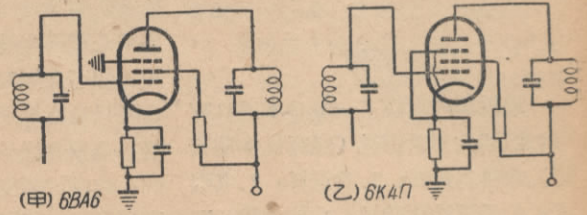
圖 4 中頻放大級綫路圖
