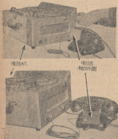
图1 电话检听器
