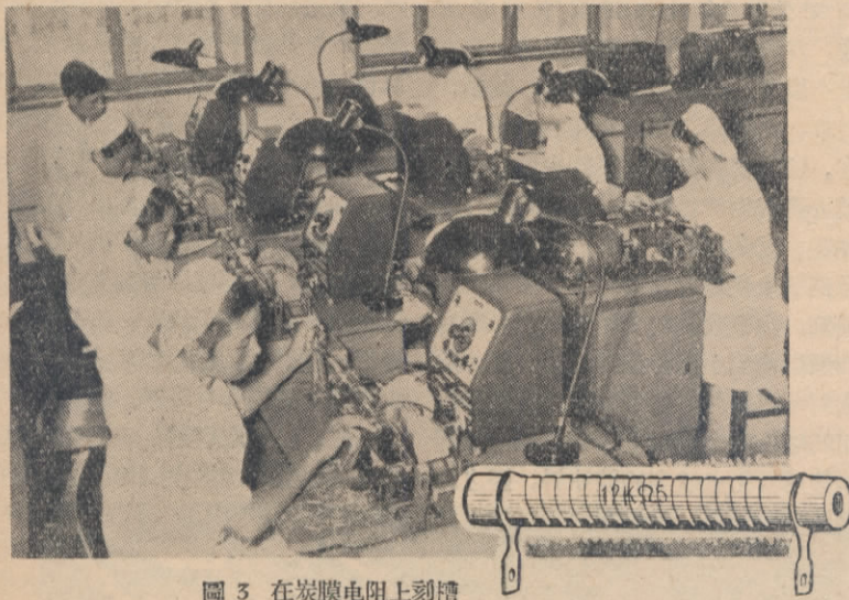
圖 3 在炭膜電阻上刻槽
