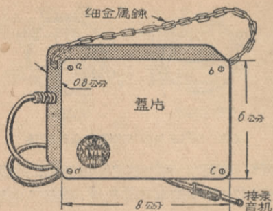
图2 电话检听器外形
